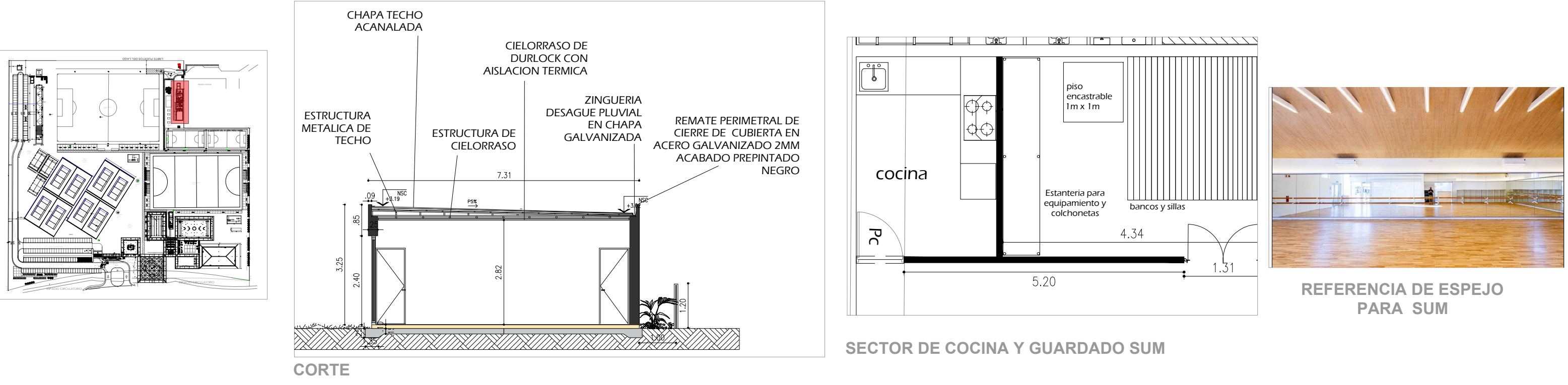
PLANTA
